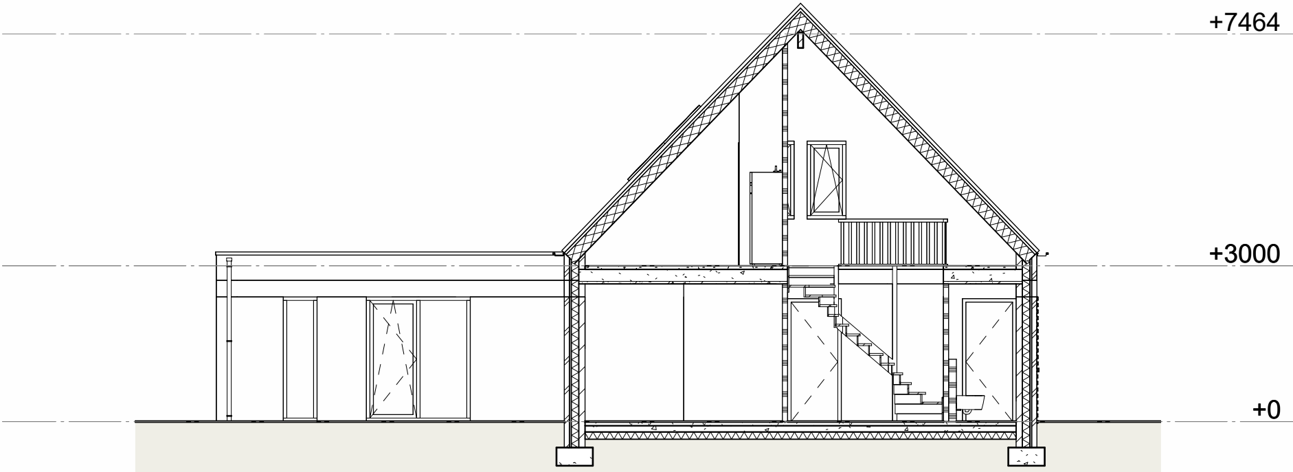
Doorsnede 1 : 100
