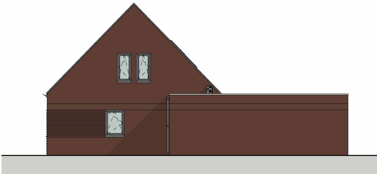
Rechterzijgevel 1 : 100
